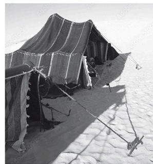
Cet habitat nomade offre de grandes possibilités de déclinaison par un système constructif auto-portant ou maintenu par des éléments extérieurs.
